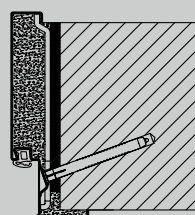
Muromvattend kozijn Diagonale bevestiging tot muurdikte 175
