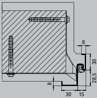
Profiel 11100
