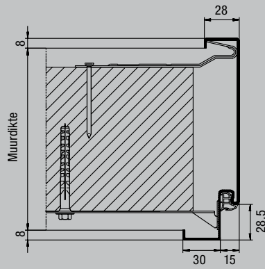
Profiel 21100
