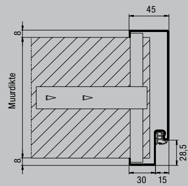
Profiel 21101
