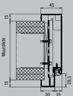
Profiel 21180 met opdek
