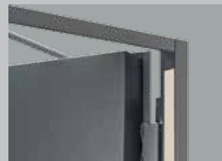
Verborgen, in hetzelfde vlak liggend brandbeveiligingsmateriaal in de zijstijlen van het kozijn (T60/T90)
