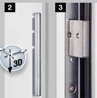
Driedimensionaal regelbare rolscharnieren voor lichtlopende deuren
