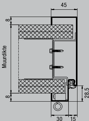
Profiel 21120
