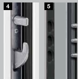
Draaigrendel met veiligheidsspennen
