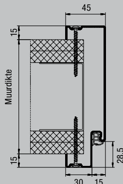
Profiel 21120 Spiegelschroefbevestiging
